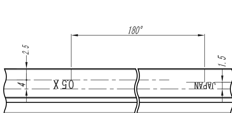
彫刻図／展開図 文字・線/太サ: 0.3
